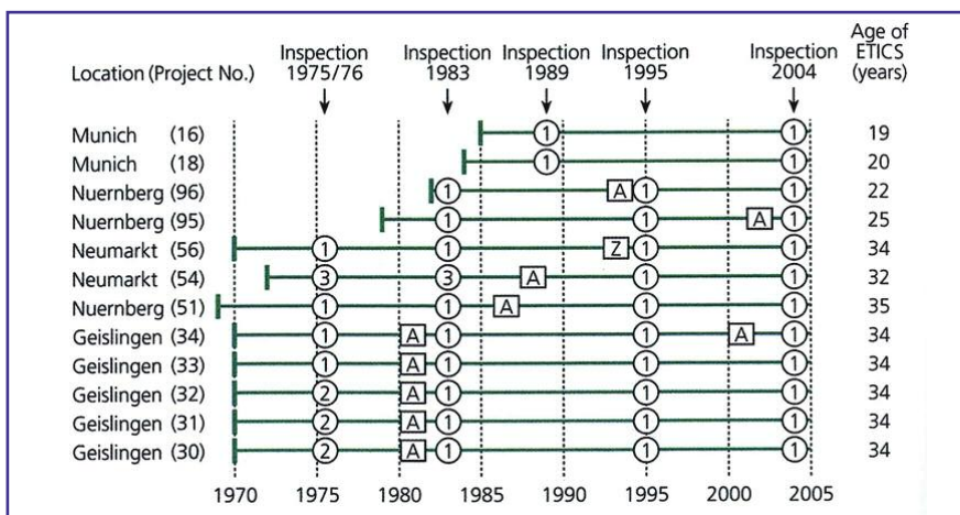
Fig. 7 - Analisi storica dei difetti rilevati su ETICS. Osservando il grafico si ha: 1 (difetti non visibili), 2 (piccole lesioni nelle zone d'angolo e vicino alle finestre), 3 (maggiori difetti: grandi distaccamenti e delaminazioni), A (nuove facciate), Z (edifici obsoleti risanati con ETICS s=4 cm).
