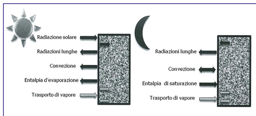
Fig. 3 - Bilancio energetico giornaliero di una parete tipo.
