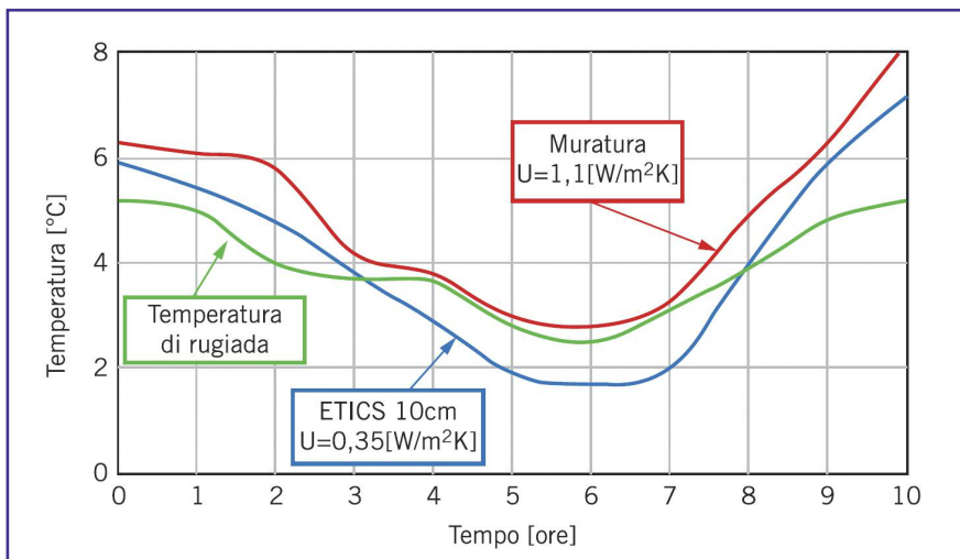
Fig. 6 - Confronto tra i profili termici superficiali di una parete leggera e massiva non isolata e la temperatura di rugiada.
