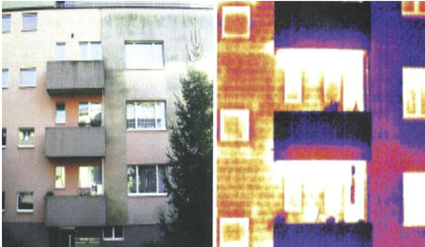
Fig. 4 - È evidente la più veloce formazione di alghe su superfici fortemente isolate.
